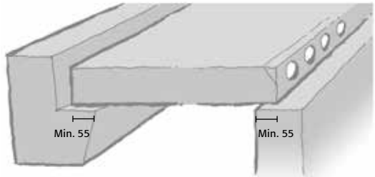
Figur: Vederlag huldæk
