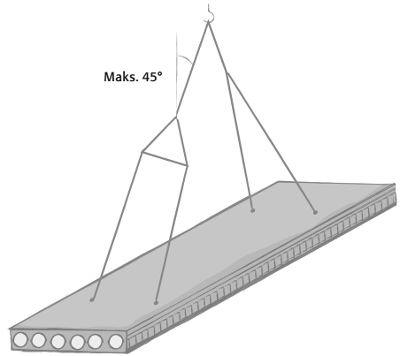
Figur: Løft huldæk
